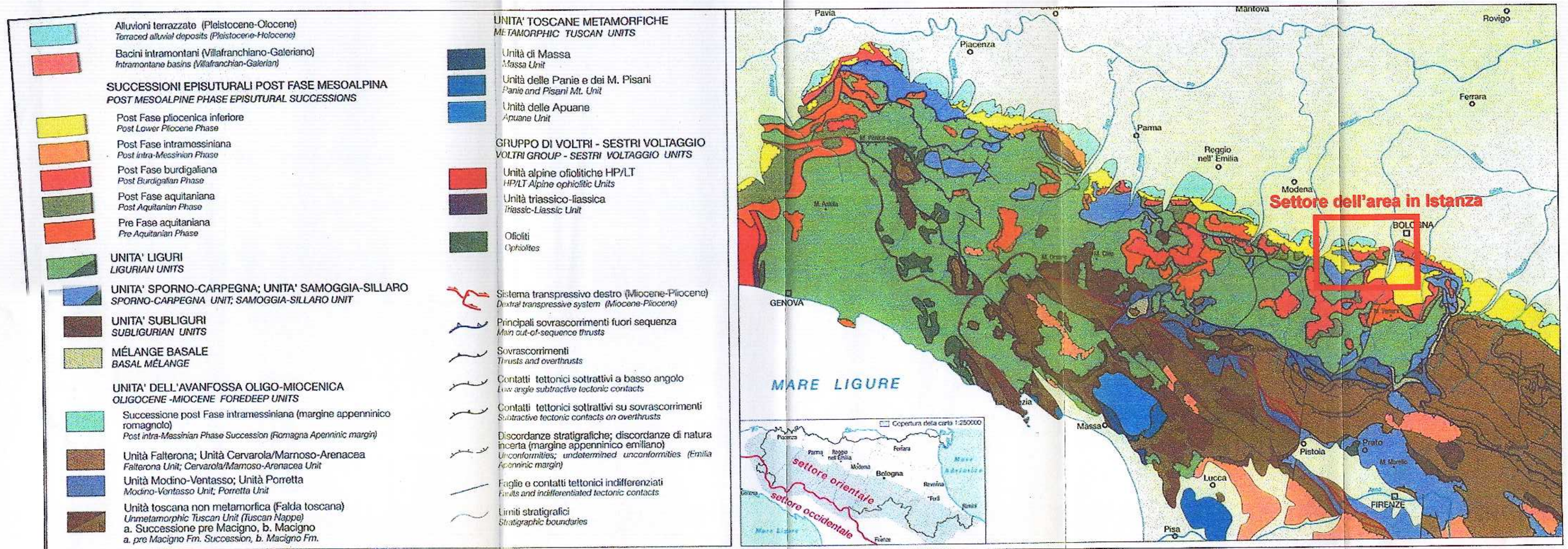
Schema Tettonico dell'Appennino Settentrionale (tratto da Carta Geol. Strutt. Dell'Appennino Emiliano-Romagnolo, Regione Emilia Romagna, 2002)
