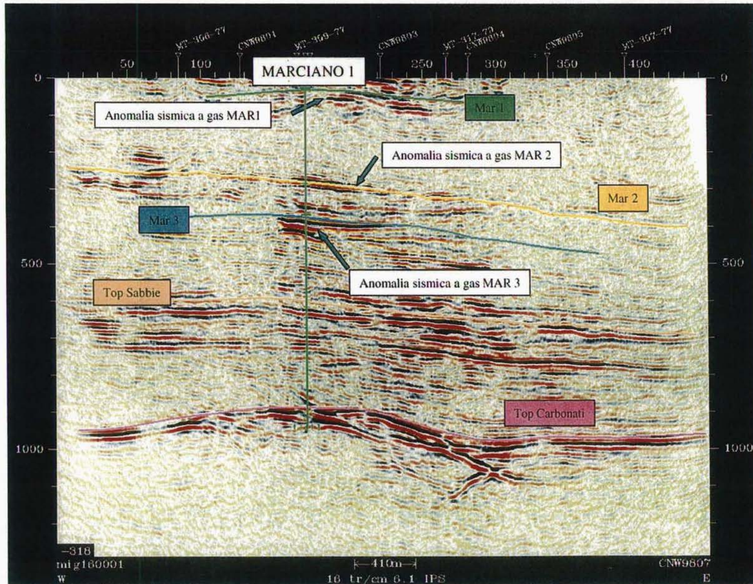
Linea sismica CNW9807
